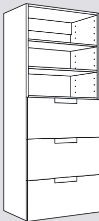
1536H x 600W x 380D 1x Cabinet Shell I/N: 0430599 1x Adj Shelves 2pk I/N: 0430838 3x Drawers I/N: 0430710 bundle0635
