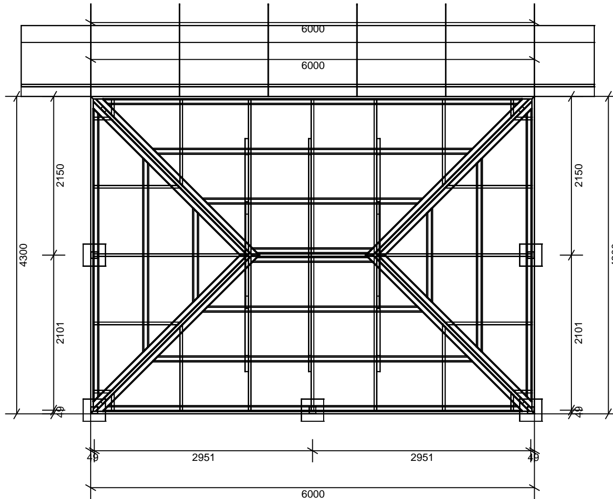
PLAN 1:50
