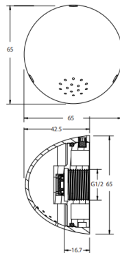
Overall Dimensions 65mm (w) x 42.5mm (d) x 65mm (h)
