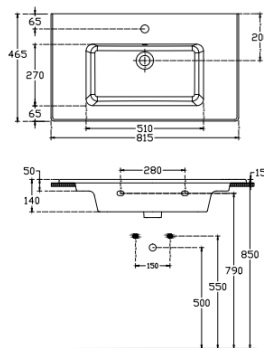
Overall Dimensions 815mm (w) x 465mm (d) x 140mm (h)
