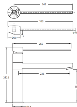
Overall Dimensions 54mm (w) x 272mm (d) x 252.5mm (h)
