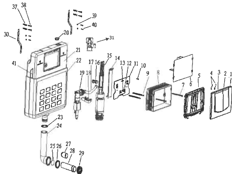
009 cistern body
